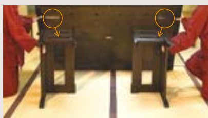
④天板裏のサンを脚の固定用枠に収めます。 グラツいたり金具が壊れる心配がないのはこの構造のためです。
