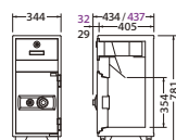
PS-20E ¥191,000 (税別) 外寸: W344×D437×H781 (mm)
