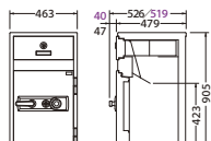
PS-50E ¥387,000 (税別) 外寸: W463×D519×H905 (mm)
