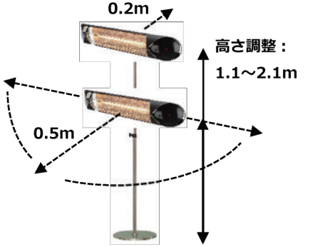
図：スタンド設置の場合の離隔距離
