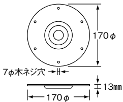
No.203 170φ 丸鉄板木ネジ ¥2,100
