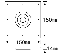
No.202 150×150 木ネジ8ヶ穴 ¥1,700
