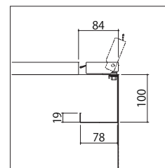
配線トレー寸法
