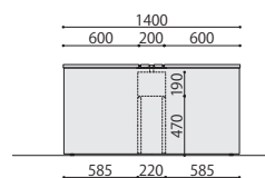
基本タイプ
