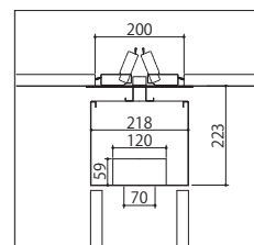
配線トレー内寸図
