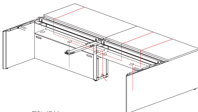
配線レイアウト
