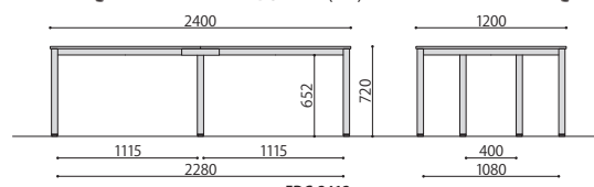
FDC-2412
