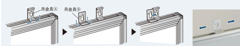
UM34N ¥39,100 板面寸法／W1210×H910 有効寸法／W1170×H870 粉受長さ／L=1200
