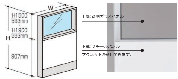
直線 上部ガラスパネル(スチールタイプ)
