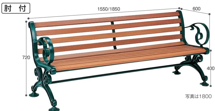
ベンチスワール®(1800 肘付)
