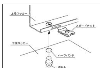
TKM-5の取付方法
