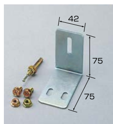
TKU-2 ¥1,600 1166 壁固定金具
