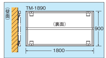
取付け図・構造図
