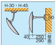
H-30・H-45 取付け図・構造図
