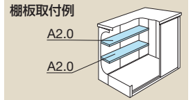
棚板取付例 (単位：mm)
