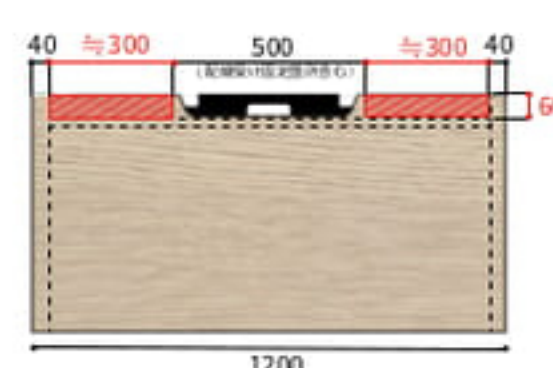
クランプの取付可能範囲は配線切り欠きの両サイドそれぞれ約300mmの範囲です
