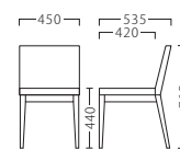
ケルプイスBR 11534-A C/レザー・ゼラファイト・プロL-6483 塗装色：BR
