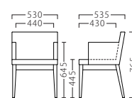
ケルプアームイスBR 11535-A C/レザー・ゼラファイト・プロL-6483 塗装色：BR
