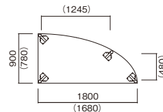
W1800×D900×H700
