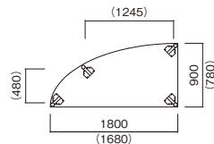
W1800×D900×H700
