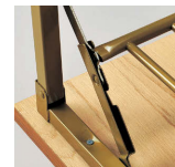
■クランク式折りたたみ機構 使用時の脚部ロックを手動で行います。
