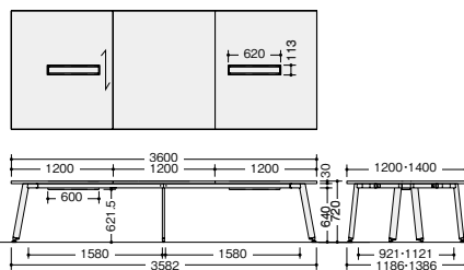
KDX3612H-□ KDX3612-□ (配線ボックスなし) KDX3614H-□ KDX3614-□ (配線ボックスなし)
