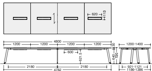
KDX2412H-□ KDX4812-□ (配線ボックスなし) KDX4814H-□ KDX4814-□ (配線ボックスなし)
