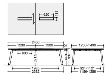
KDX2414H-□ KDX2412-□ (配線ボックスなし) KDX2414H-□ KDX2414-□ (配線ボックスなし)
