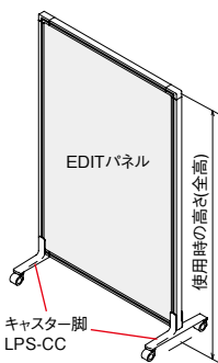
【基本パターン】 EDIT パネル × 1 枚 キャスター脚 × 2 個
