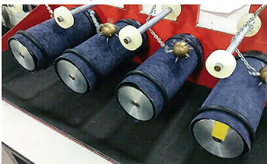
ICI 形メース試験機 スナッグ試験
