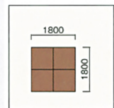
※写真のレイアウト構成 / ST-9430H×1, ST-9280H×2, ST-9130H×1
