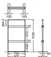
FB-1508BOX (K)
