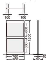
FB-1508CP (H)
