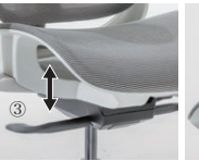
①座面調整レバー ②ロックレバー(4段階) ③座面昇降レバー ① Seat adjustment lever ② Rocking lever (4 levels) ③ Seat elevation lever
