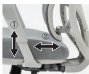
① ロッキングレバー (4段階) ・座面高さ調整 ② 座面前後調整レバー ① Locking lever (4 levels), Seat height adjustment ② Seat forward/backward adjustment lever
