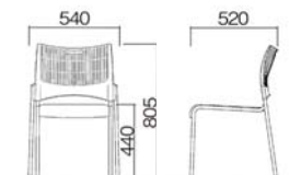
クリスト DMC21 W540×D520×H805 (SH440) 4.8kg
