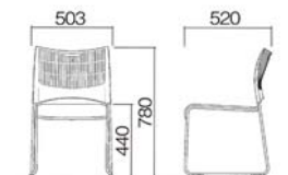
クリスト DMC20B W503×D520×H780 (SH440) 3.6kg
