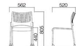
クリストOBP DMC24C-OBP W562×D520×H805 (SH440) 4.9kg ●海洋プラスチック再生樹脂
