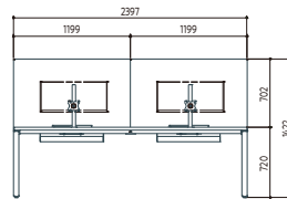
シングルモニターアーム 無段階で高さ調整/ 首振り角度調整が可能。 支柱高さ: 385mm VESA規格: 75×75/100×100 推奨モニターインチ: ~30インチまで 耐荷重: 10kg
