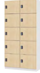
AYSL2-5(2列5段10人用) W900 D455 H1800 主材/スチール
