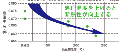
熱処理温度と熱伝導率 引用：豊野まなみ他：第8回 日本木材学会大会研究発表要旨集 71 (2008)
