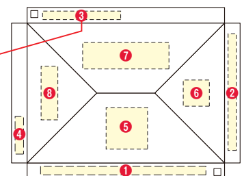
DX45 (3.0×4.5m) 展開図
