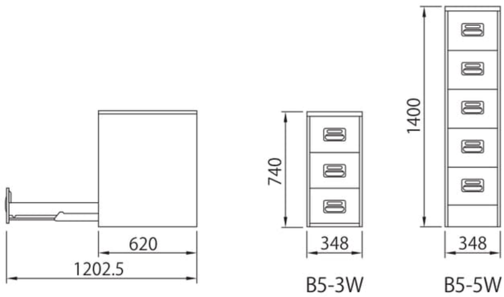
脇机型3段 B5-3W ¥77,900 引出し内寸法/W280×D562×H212 質量/32.5kg B5W仕切板6枚
