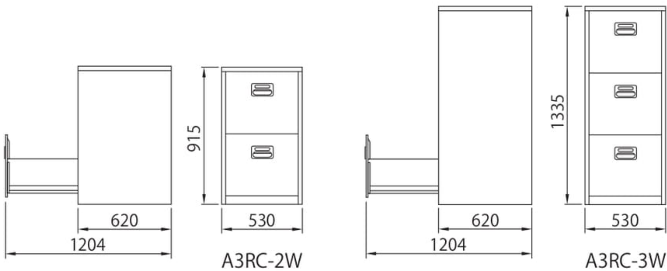
A3RC-2W ¥125,400 引出し内寸法/W460×D561×H392mm 質量/44kg A3RCW仕切板4枚付
