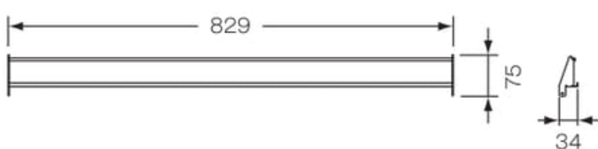
前後フレーム
