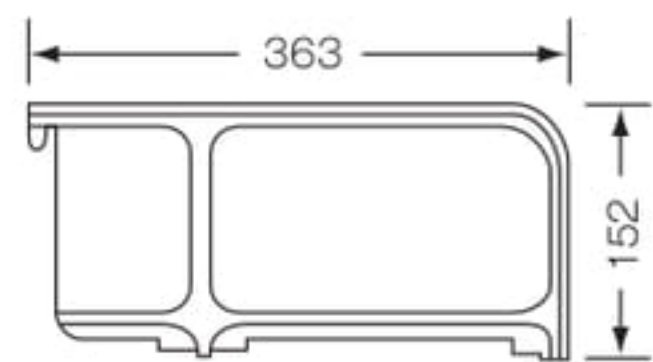
クロスタテ仕切板
