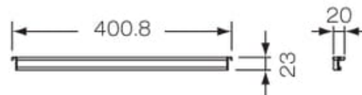
サイドフレーム(2本1組)
