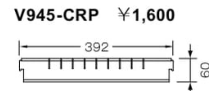
クロスタテ仕切板
