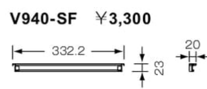
前後フレーム
