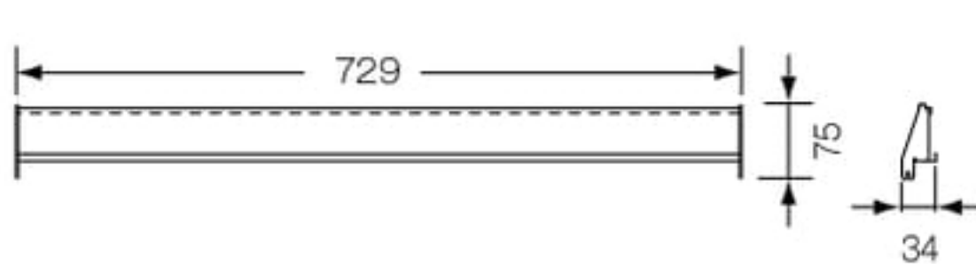
前後フレーム
