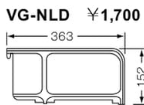
自在仕切板
