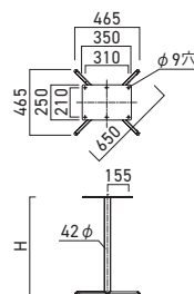
GM-GL 650L (ゴールド)
