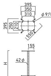
GM-GL 550L (ゴールド)
