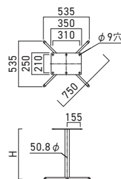
GM-GL 750L (ゴールド)
