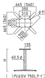
GV-PO 750L・900L (研磨仕上げ)
