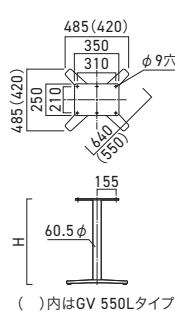
GV-PO 550L・640L (研磨仕上げ)
