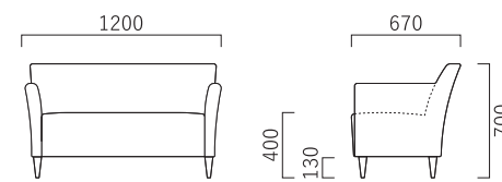
2人掛け サイズ: W1200×D670×H700×SH400mm
