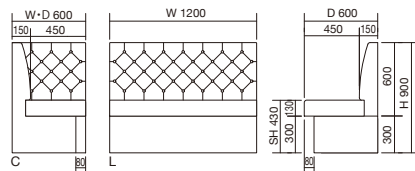
3型C 例: W600×D600×H900・SH430mm 台輪: グレー
