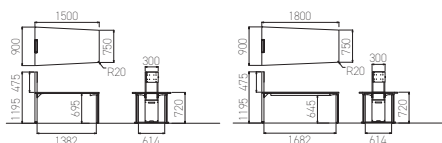
SJ脚テーパ天板1590
