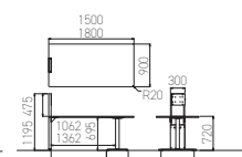
一本脚角天板1590_1890
