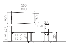
一本脚テーパ天板1590/1890
