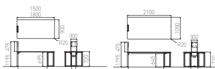
ループ脚角天板1590/1890
