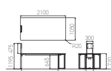
ループ脚角天板2110
