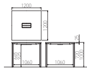
SJ□-1212NA/HA (+配線ボックス付)
