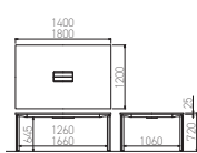
SJ□-1412NA SJ□-1812NA (+配線ボックス付)
