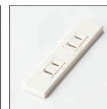
2口コンセント 2口コンセント (WHT天板のみ) W110×D24×H6.5mm コード長さ1970mm
