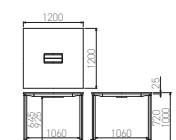
SJ□-1212NC/HC (+配線ボックス付)
