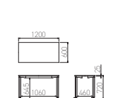
SJ□-1260NC
