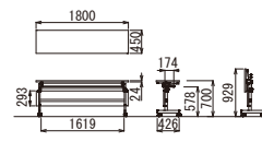
YST-1845 幕板付き
