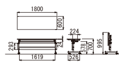
YST-1860 幕板付き
